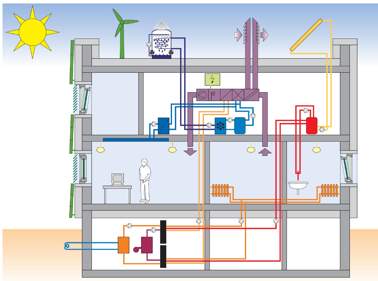
Bild 2 — Inhalt und Umfang von DIN/TS 18599-10 (schematisch)
